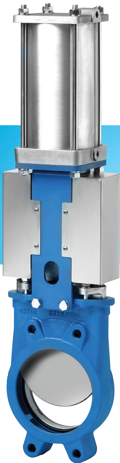
EX Unidirecional DN 50 – DN 1200 ferro fundido / aço inoxidável
