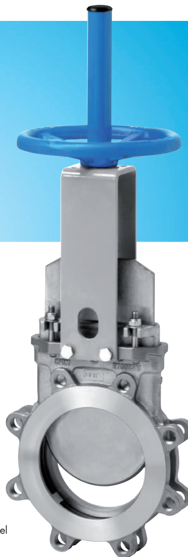
ET Unidirecional MSS SP-81 DN 50 – DN 900 aço inoxidável
